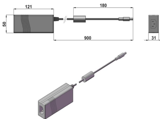
121(L)×50(W)×31(H) mm 3 , 0.3kg
